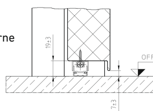
przekrój skrzydła z uszczelką opadającą
